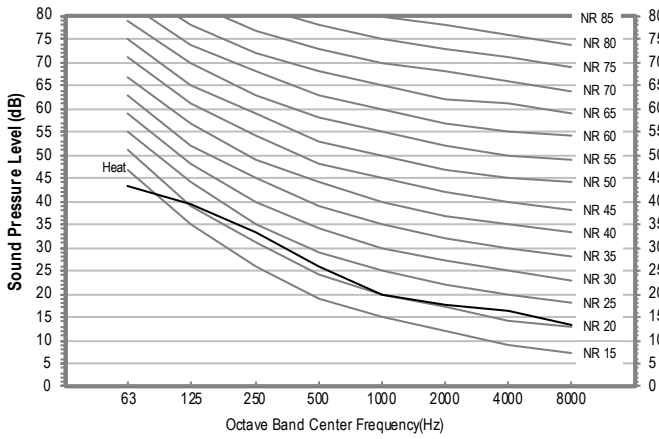
1) AE160ANYDEH/EU
